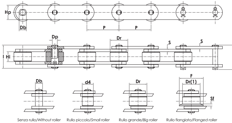
Senza rullo/Without roller Rullo piccolo/Small roller Rullo grande/Big roller Rullo flangiato/Flanged roller
